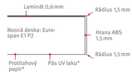
Model 100 / 1,5
